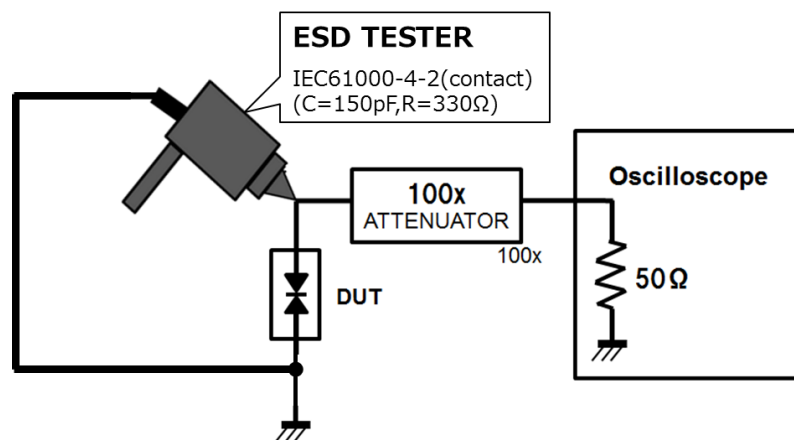
Fig. IEC61000-4-2 (Contact)
